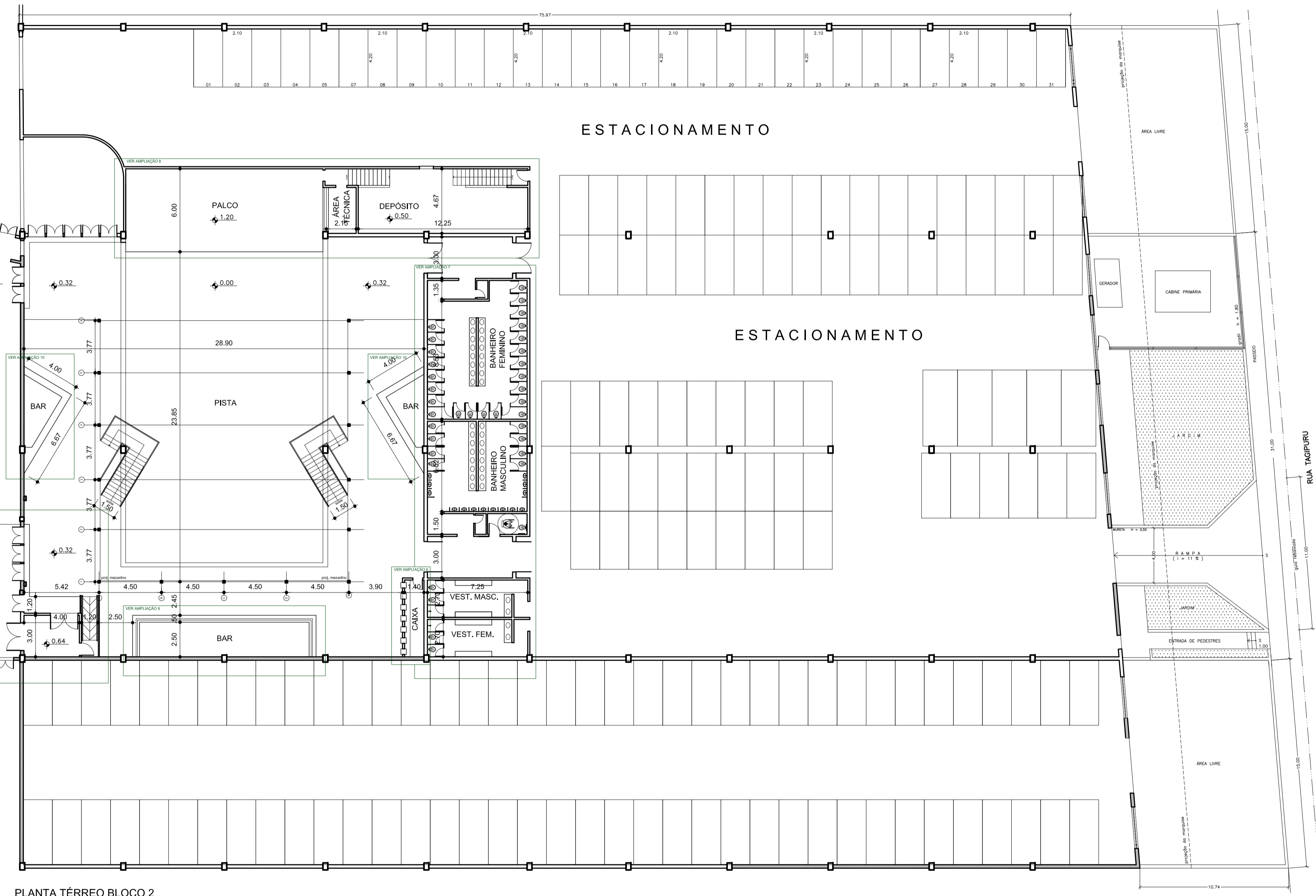
PLANTA TÉRREO BLOCO 2 esc 1:200
