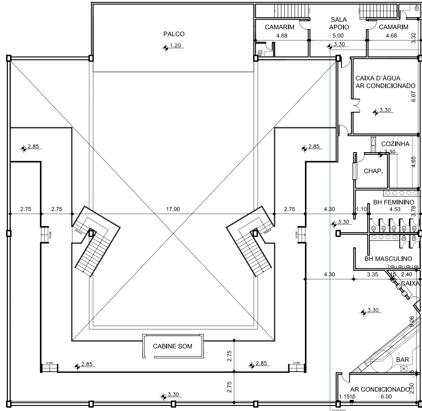
PLANTA MEZANINO esc 1:200
